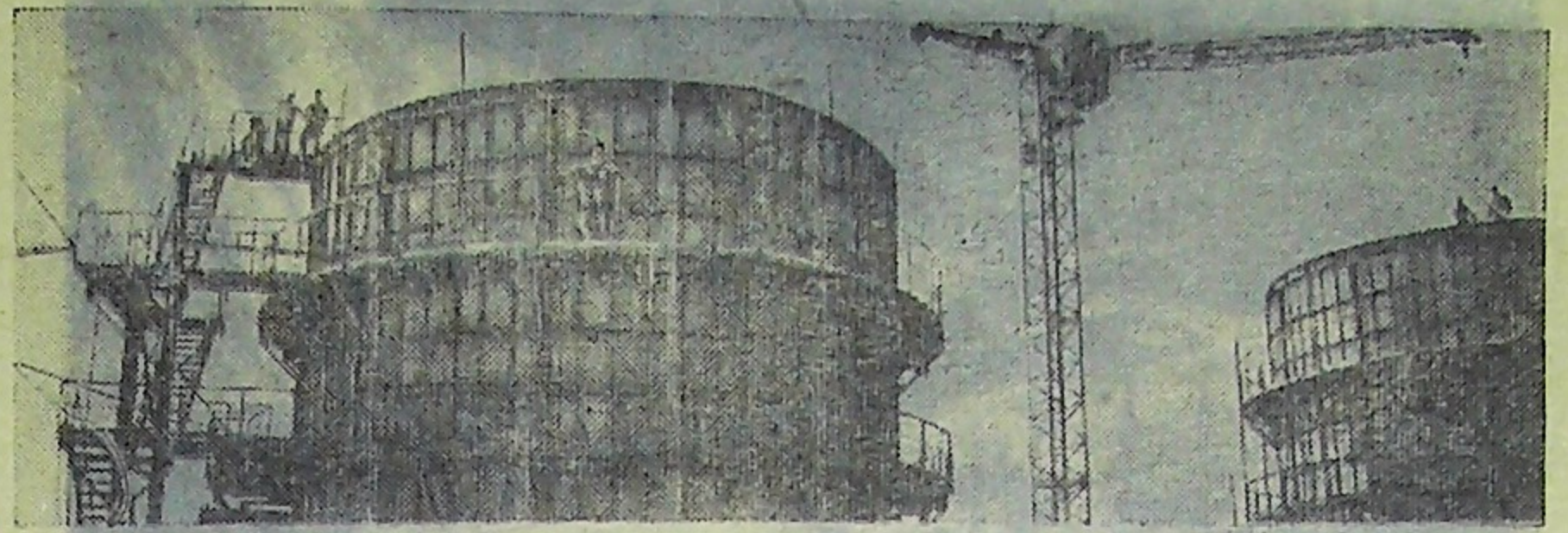
Первая очередь Башкирского биохимического комбината—пусковой объект этого года, Всесоюзная ударная комсомольская стройка. Уже в будущем году предприятие, которое сооружается близ Уфы, должно выработать 60 тысяч тонн кормовых дрожжей. На снимке: сооружаются емкости цеха сушки. Фото В. Воюга (Фотохроника ТАСС)
