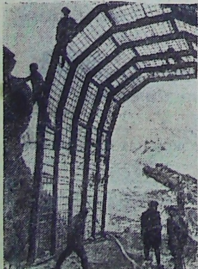
В верхнем течении реки Вахи на высоте 1110 метров будет сооружена крупнейшая в Средней Азии Рогунская ГЭС. На снимке: установка каркаса входного портала дренажного тоннеля.
