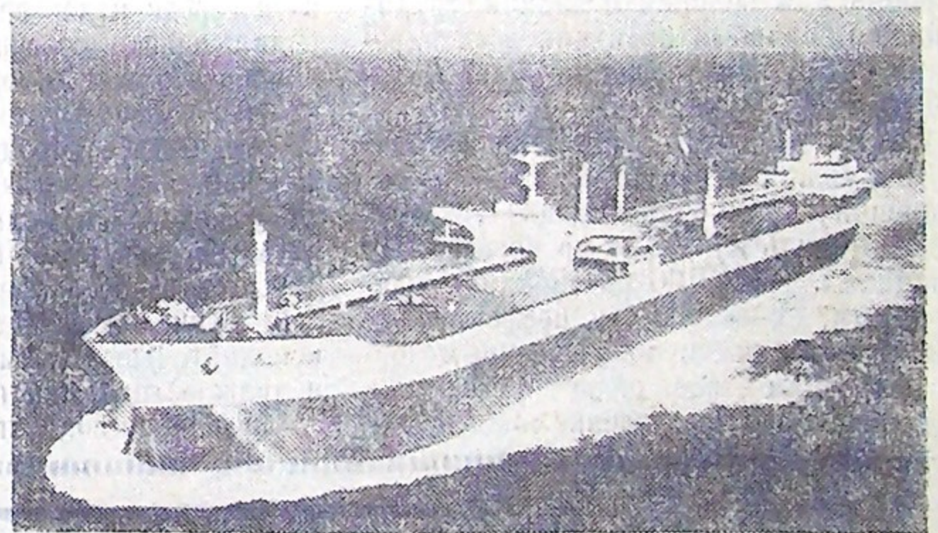
Крупнейший в мире танкер «Идэмиду-мару» отправился в свой первый рейс в Кувейт. Уникальное судно водоизмещением 210 тысяч тонн, длиной 342 метра, шириной почти 50 метров построено в Японии. Управление гигантом полностью автоматизировано, команда состоит из 32 человек.
