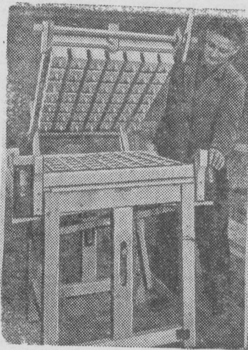
Воронежская область. Коллектив Острогосского мотороремонтного завода приступил к производству опытной партии станков для изготовления торфоперегнойных горшочков-лубиков. Этот станок сконструировал бригадир строительной бригады колхоза имени Димитрова И. А. Насимов.
