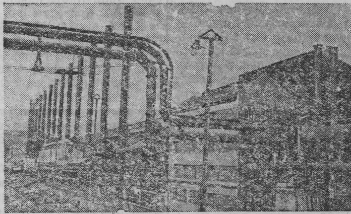
Мартеновский цех Кузнецкого металлургического комбината имени Сталина.
