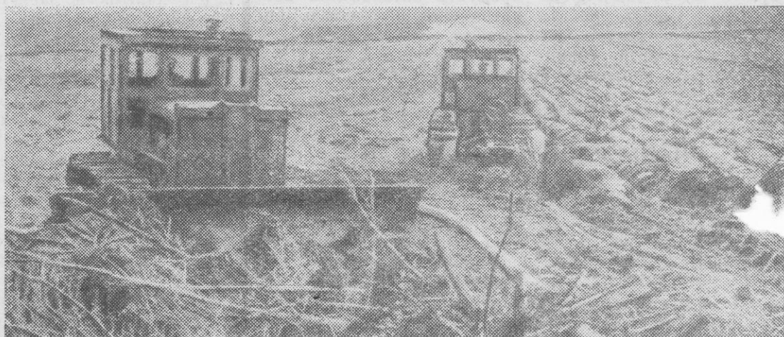
На снимке: механизаторы Иркутского треста по освоению новых земель ведут раскорчевку и глубокую вспашку отвоеванных у тайги земель, чтобы колхоз имени Ленина и совхоз «Усть-Ордынский» могли выращивать на них хлеба. Фото М. Минсева.
