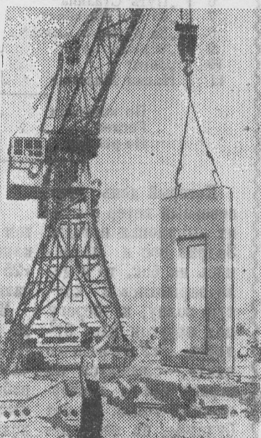
Таджикская ССР. Коллектив Сталинабадского завода железобетонных конструкций осваивает производство сборных пятиквартирных жилых домов из железобетона. Скоро начнется их серийный выпуск. На снимке: съемка с полигона сборных плит первого опытного железобетонного дома.
